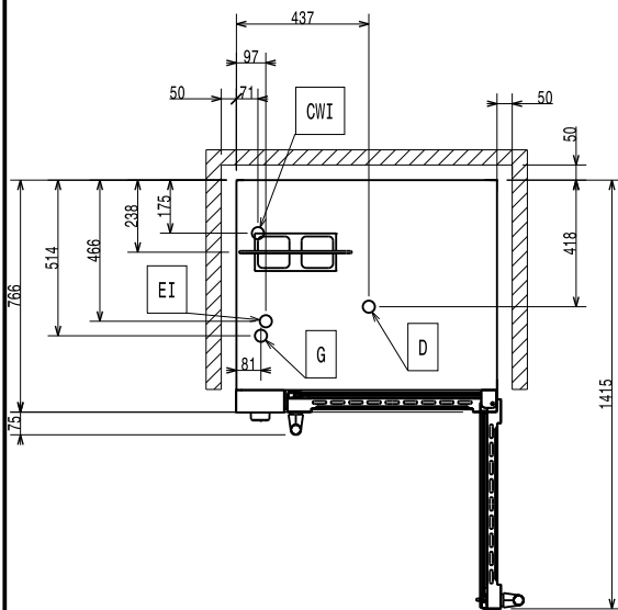
Felülnézet
